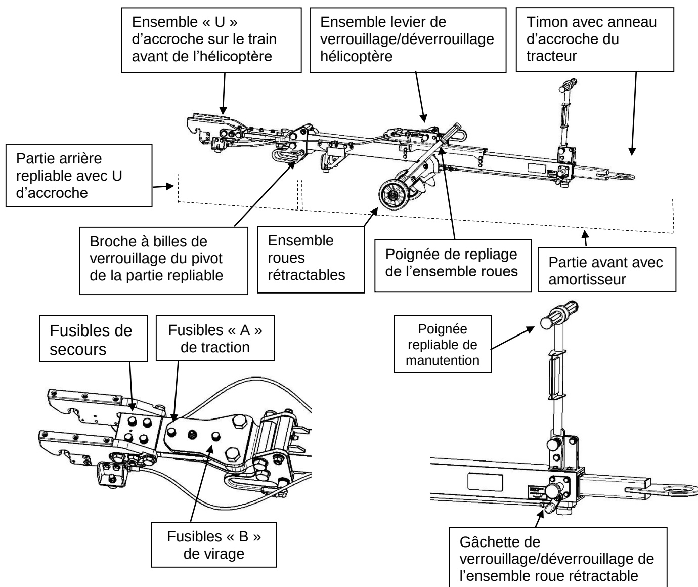
Figure 1 : barre de remorquage courte H160
