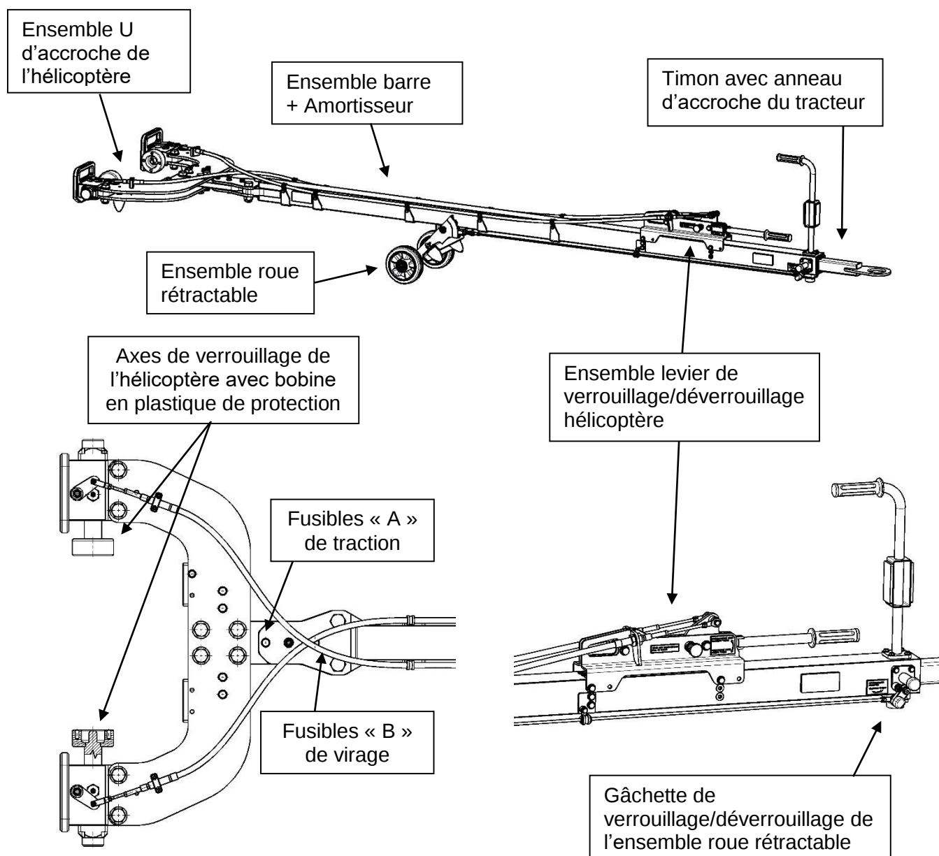
Figure 1 : barre de remorquage TB175-01
