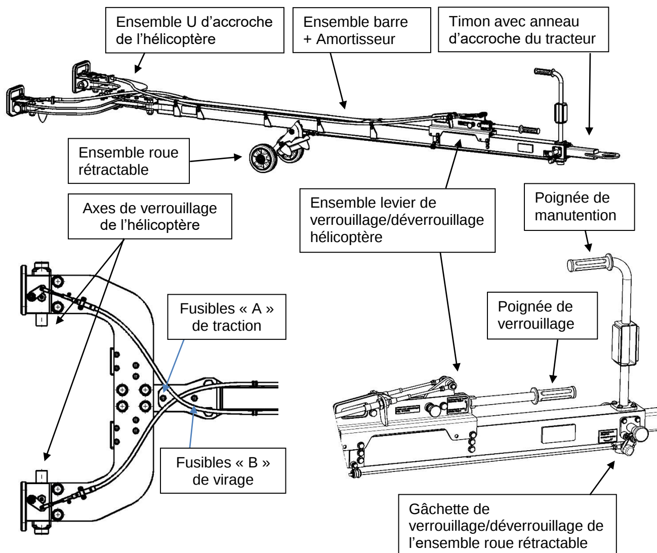
Figure 1 : barre de remorquage TB330-01
