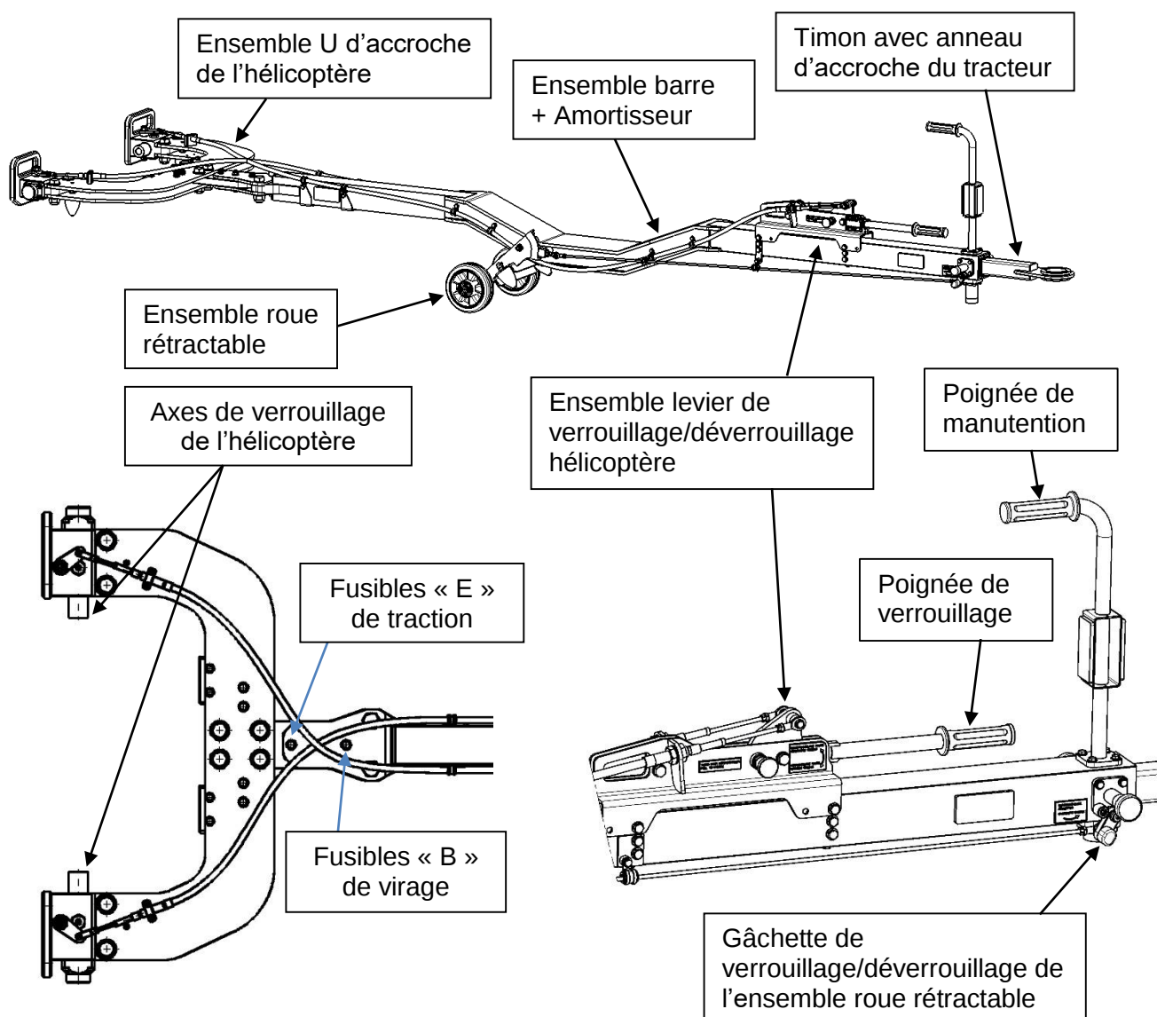
Figure 1 : barre de remorquage TB332-03
